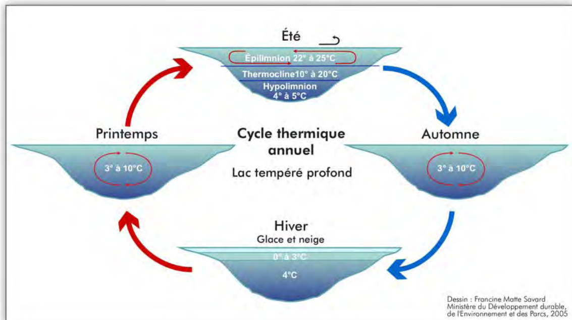
Figure 4.2 Cycle thermique annuel d'un lac
